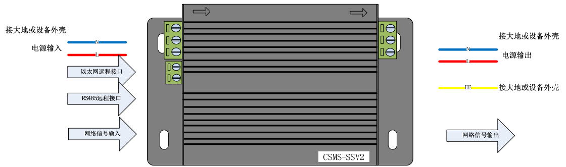
浪涌保护器安装示意图
